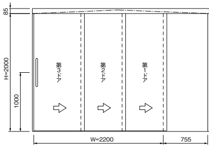
3枚連動片引き
