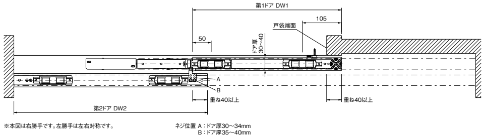
2枚連動片引き (面付型ゼンマイユニット仕様)
