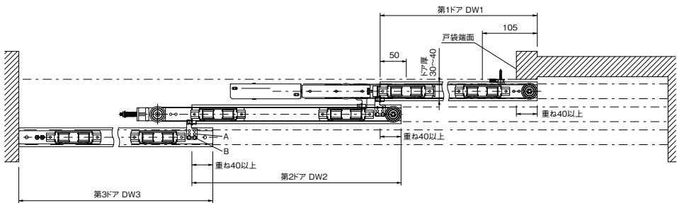
3枚連動片引き (面付型ゼンマイユニット仕様)
