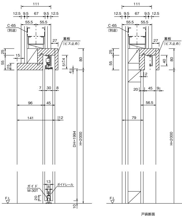
戸袋断面
