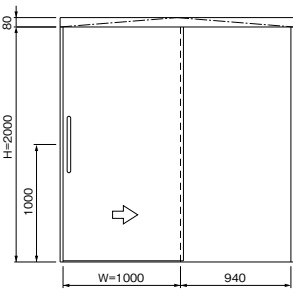
片引き
