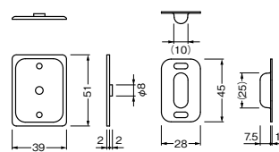
茶 白 受 ネジ止め・打込み共通金具
