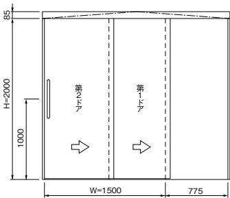
2枚連動片引き
